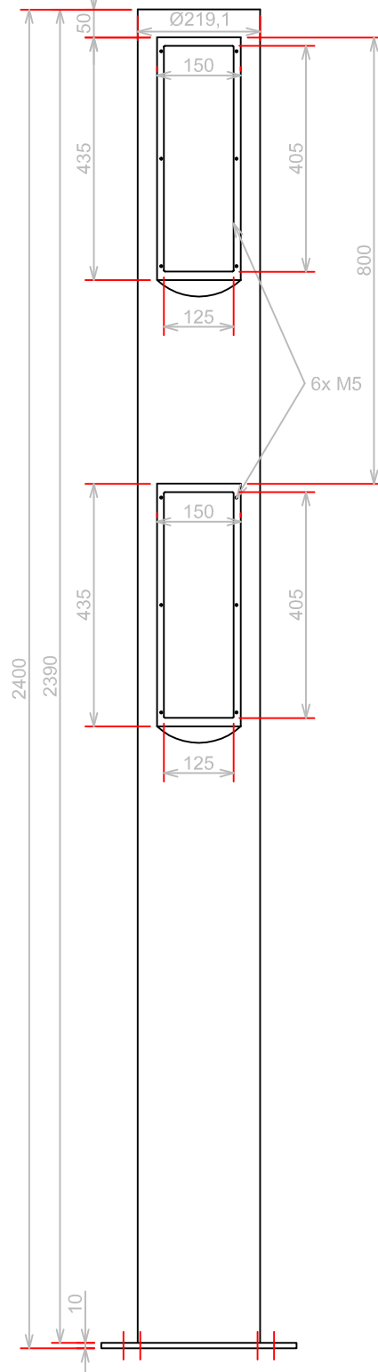
Vooraanzicht zonder alu plaat
