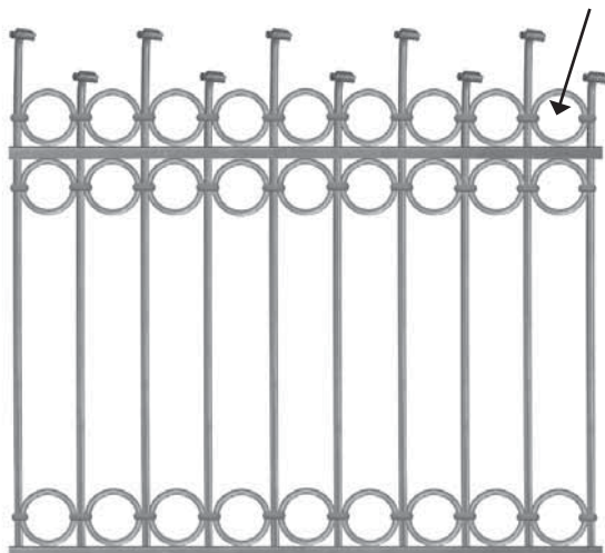
Elementi / Elements: Art.02.065.15 Art.06.032.02
